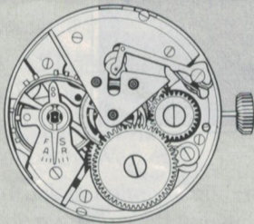
Das Werk der Chronostop · Konstruktion von 1948
